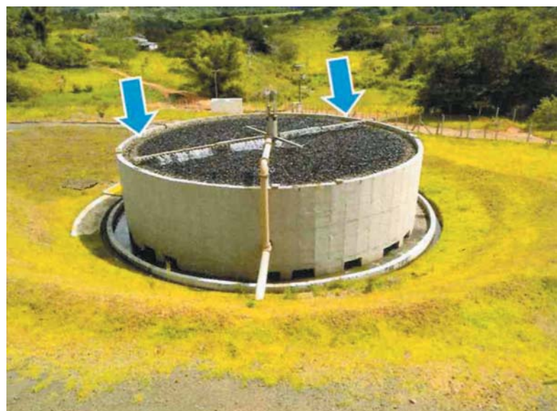
Distribuição irregular no filtro biológico percolador
